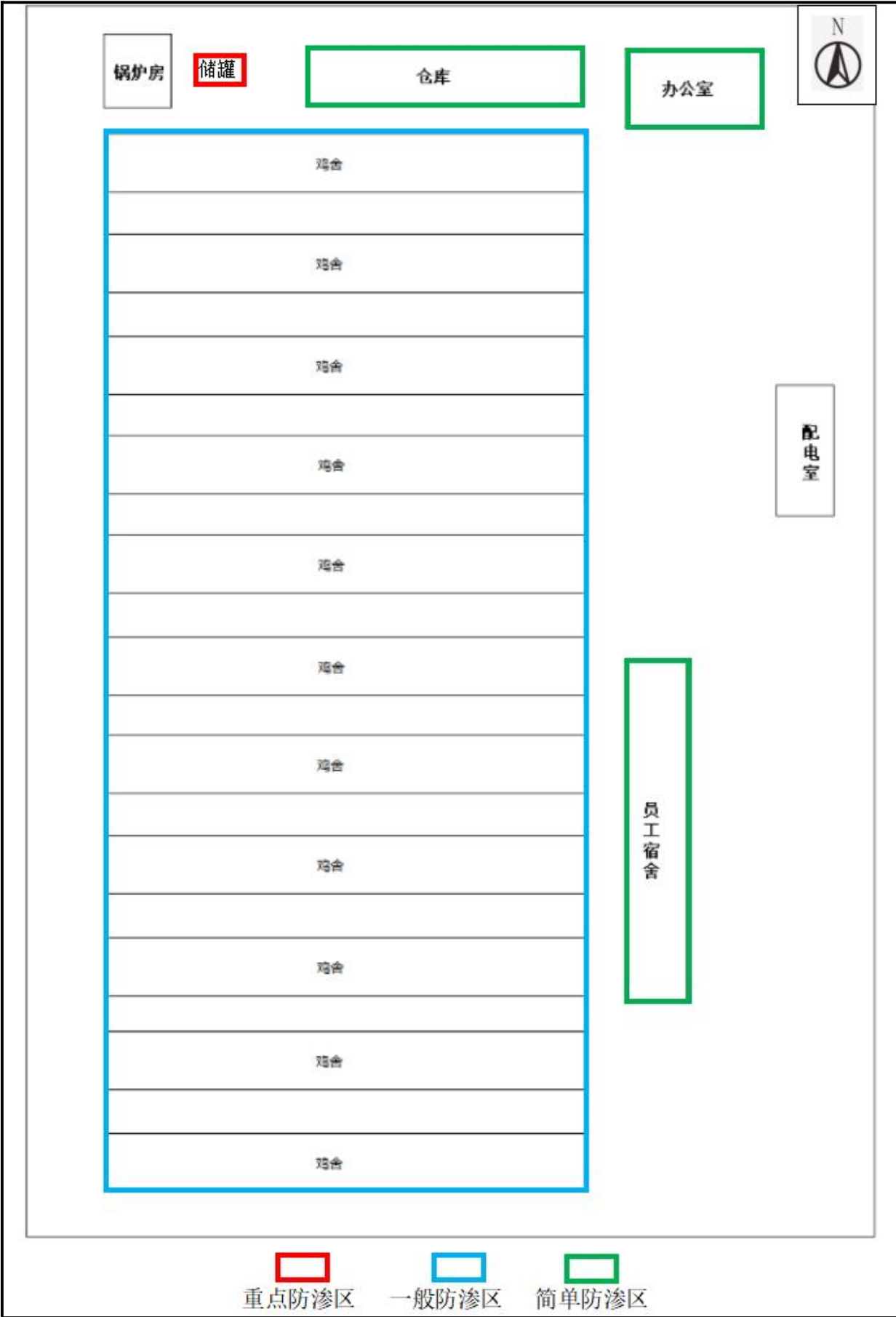
附图 5：分区防渗图
